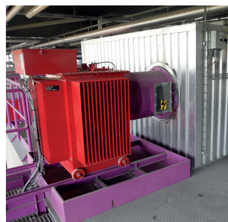
transformateur de l'électrofiltre UIOM
