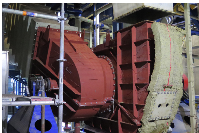
Ventilateur VT1
